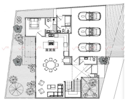
Planta Baja
